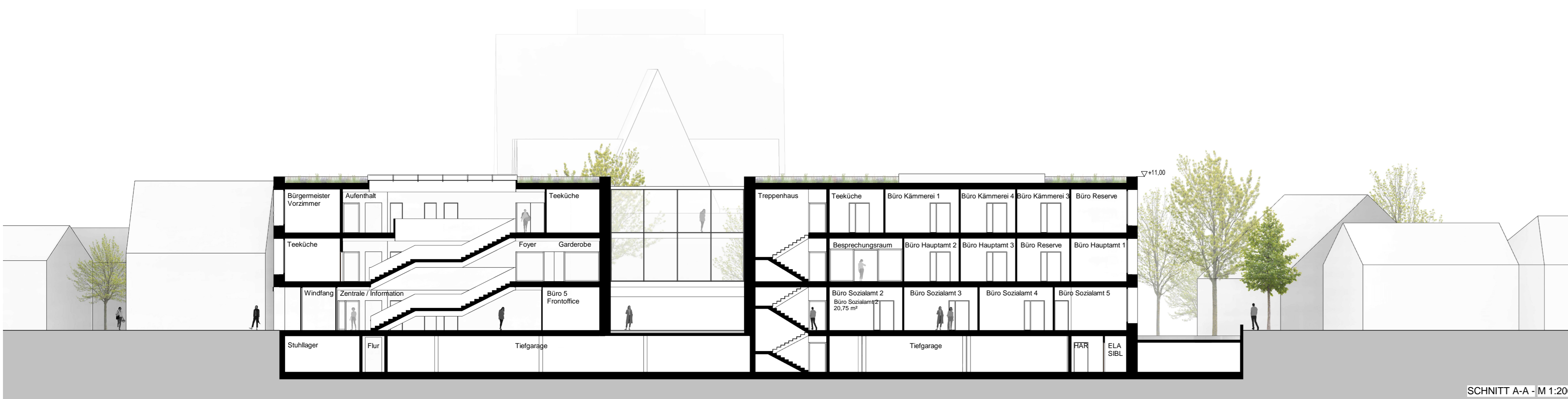
SCHNITT A-A - M 1:200
